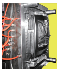
模具水路 Mold Channel
